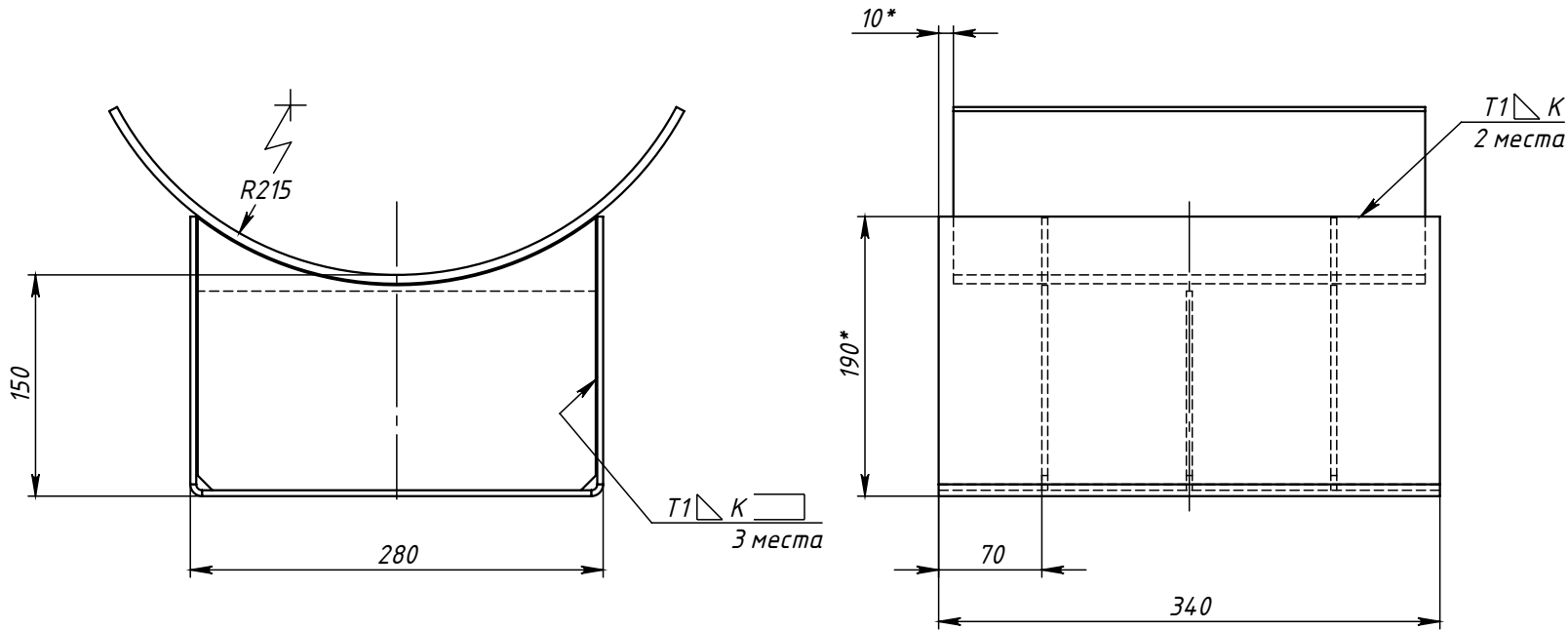
Поз.4 (Ложемент)
