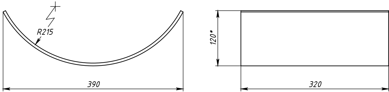
Поз.4 (Ложемент)
