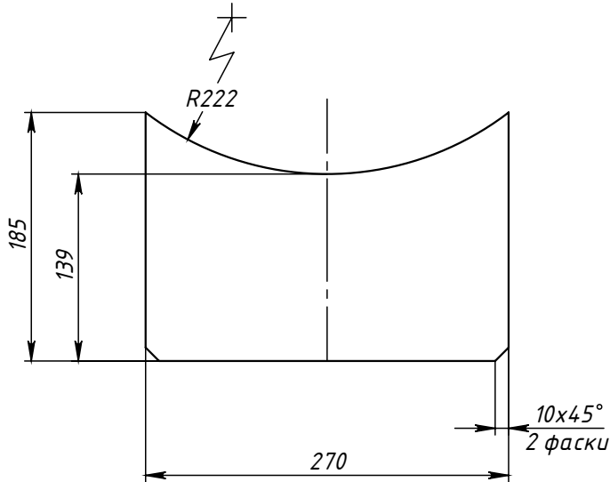
Поз.3 (Ребро)
